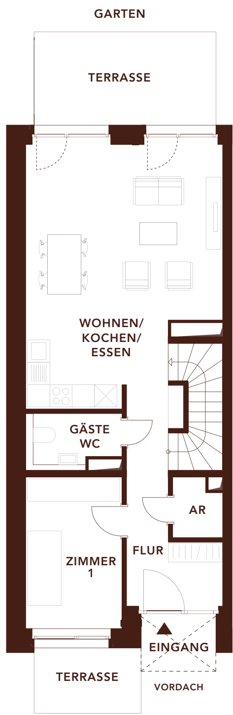
EG
